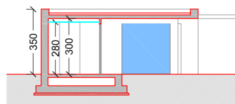
Sezione BB 1 : 200
