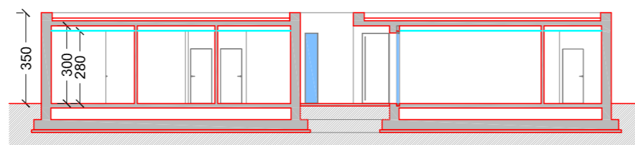
Sezione AA 1 : 200
