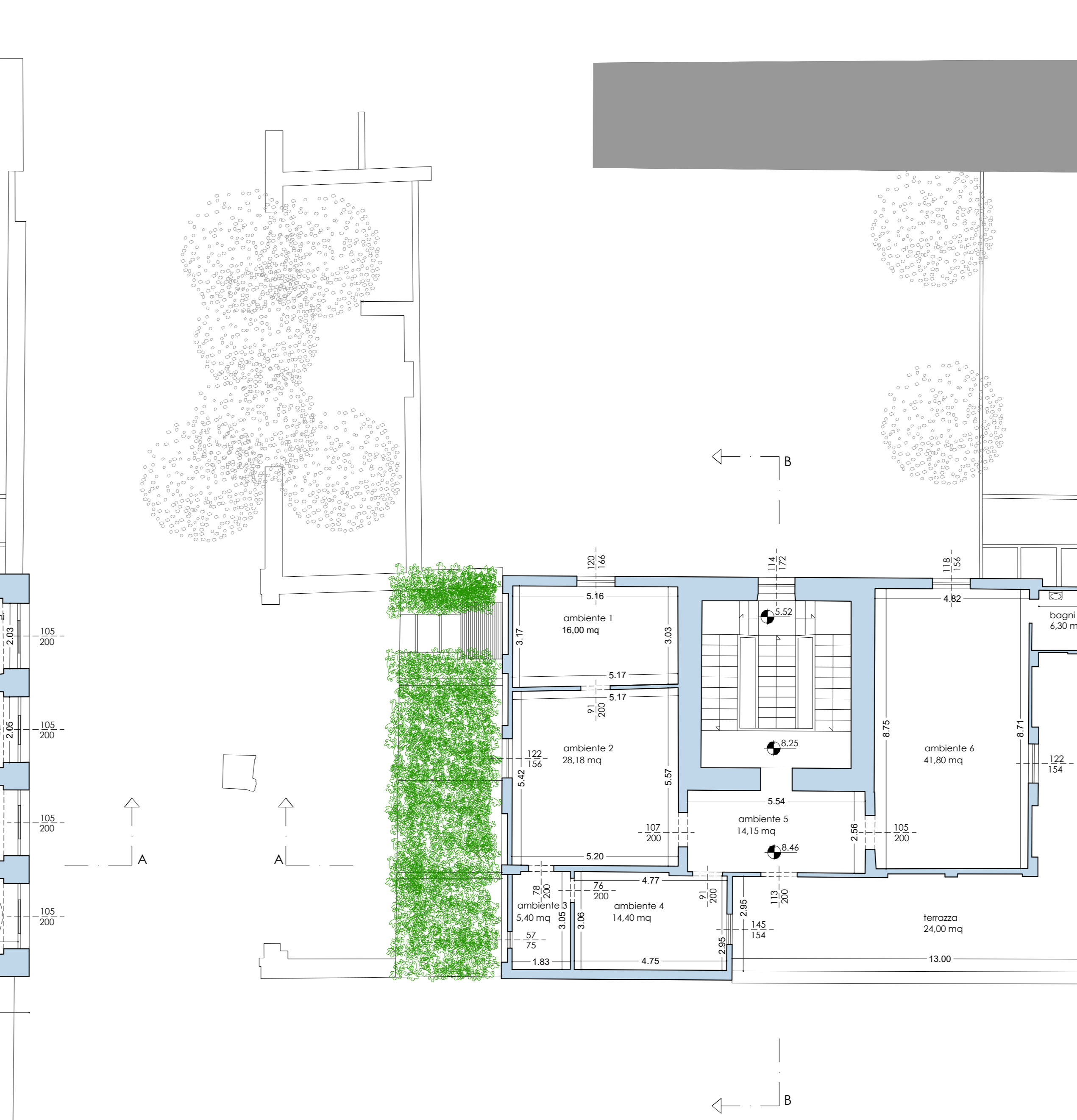
PIANTA PIANO SECONDO
