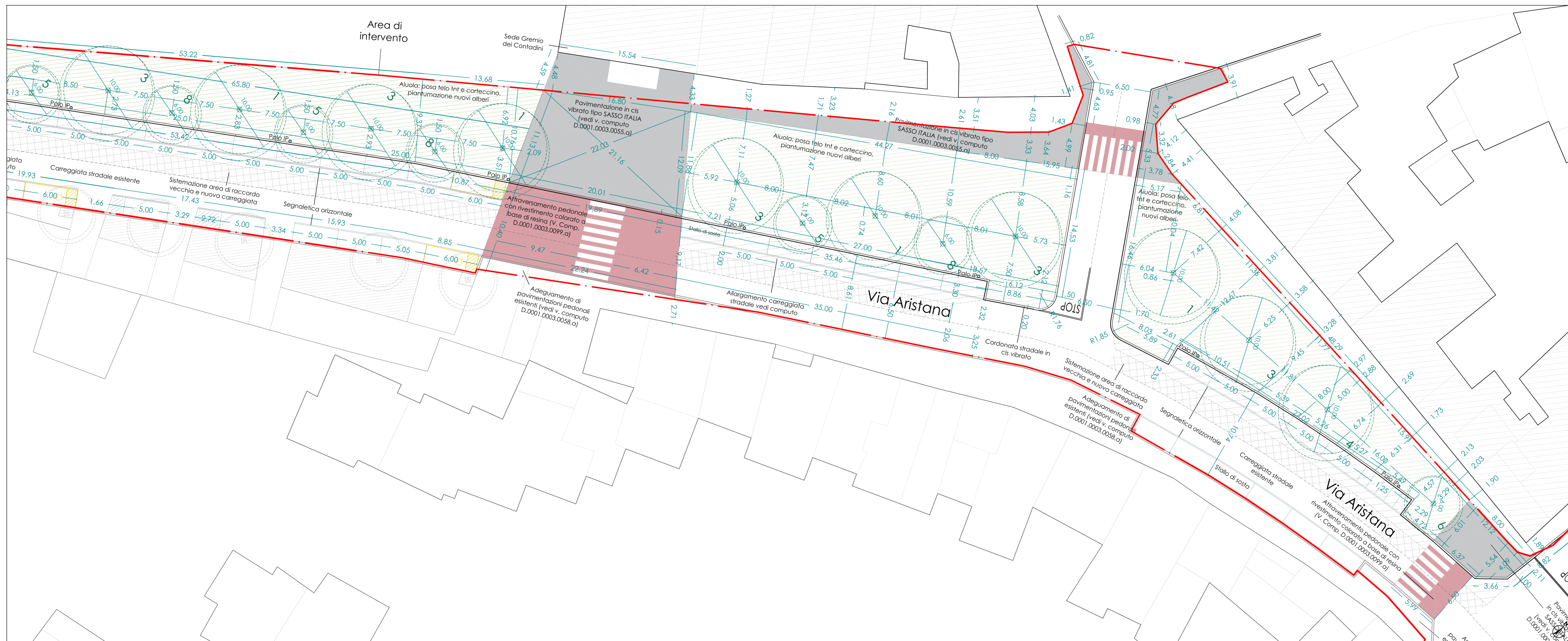
Planimetria tecnica di progetto con indicazione delle opere da realizzare Scala 1:2000
