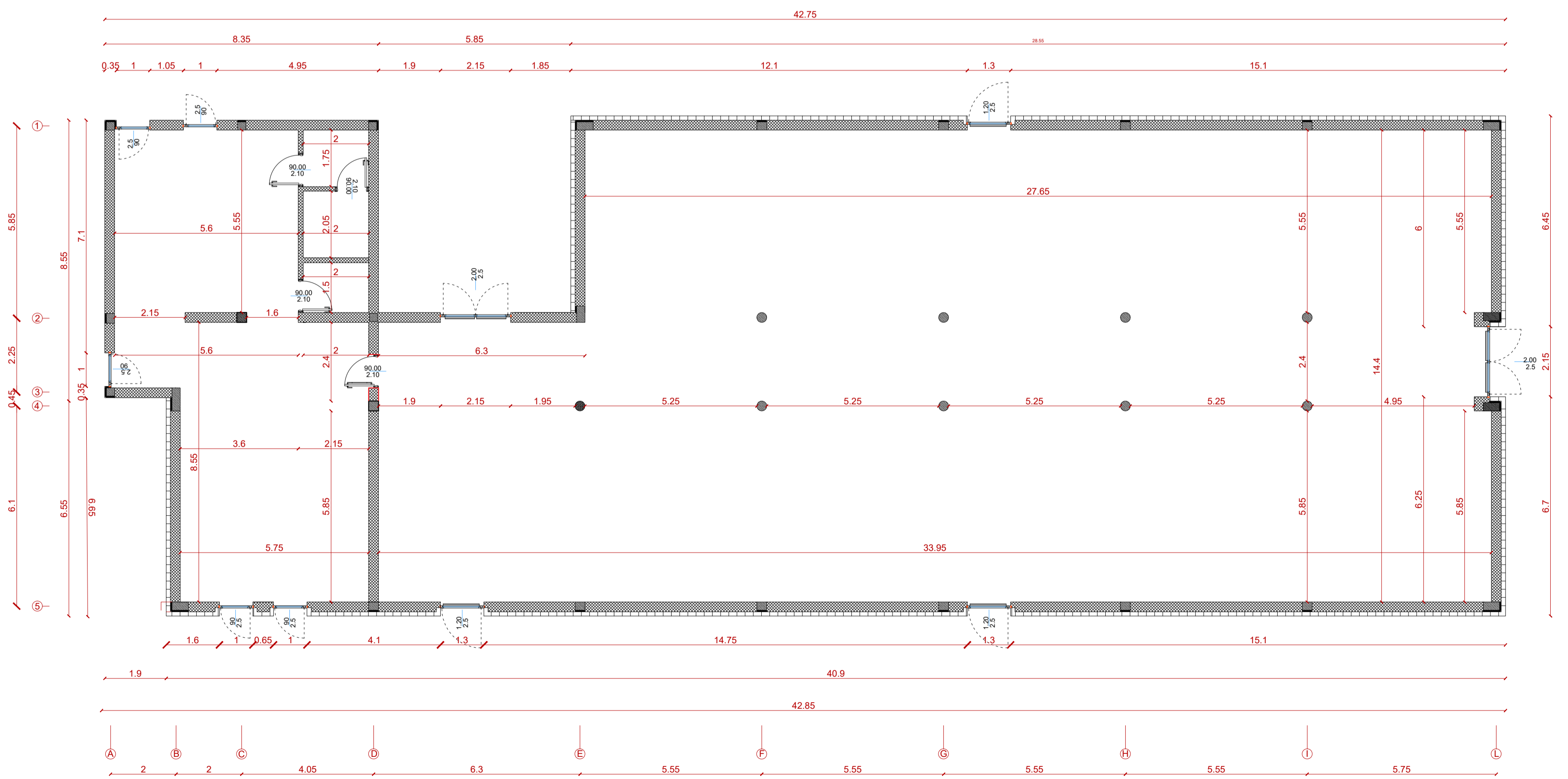
PIANTA QUOTATA
